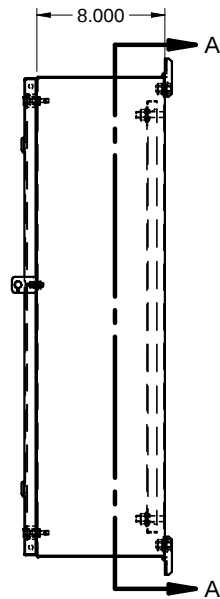
SIDE / CÔTÉ
