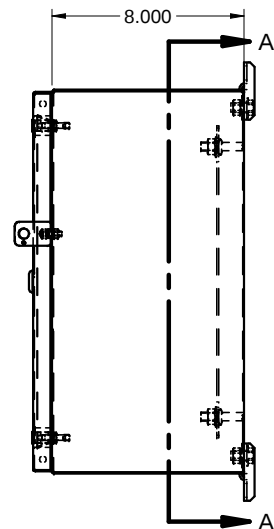
SIDE / CÔTÉ
