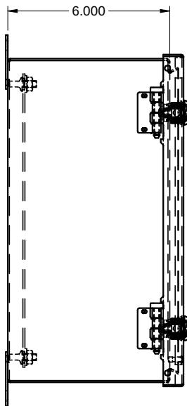
SIDE / CÔTÉ
