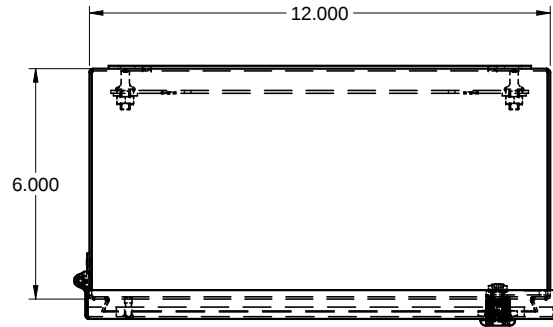
TOP / DESSUS
