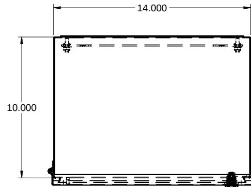
TOP / DESSUS
