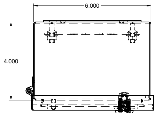
TOP / DESSUS
