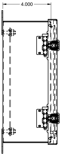
SIDE / CÔTÉ
