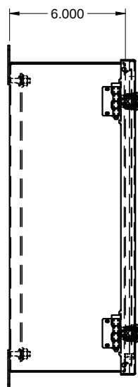
SIDE / CÔTÉ
