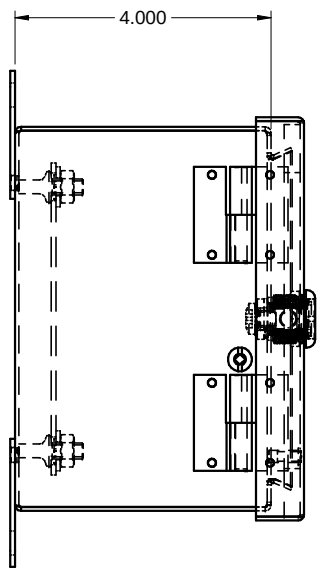
SIDE / CÔTÉ
