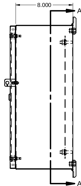
SIDE / CÔTÉ
