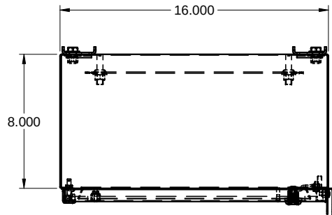
TOP / DESSUS
