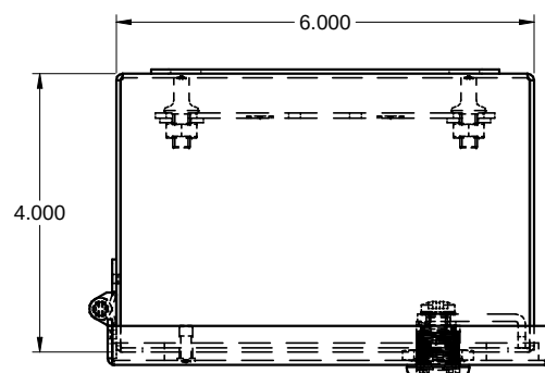
TOP / DESSUS
