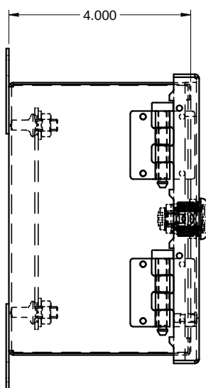
SIDE / CÔTÉ
