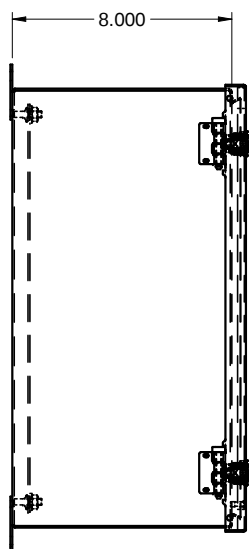
SIDE / CÔTÉ
