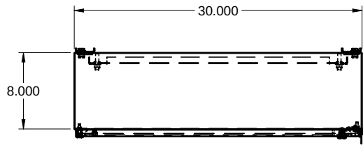
TOP / DESSUS
