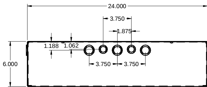
TOP / DESSUS
