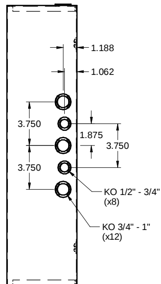
SIDE / CÔTÉ
