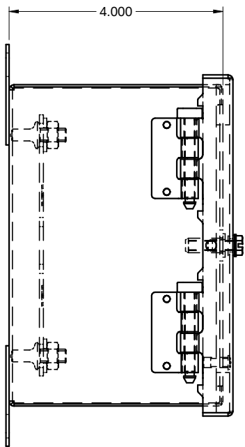
SIDE / CÔTÉ
