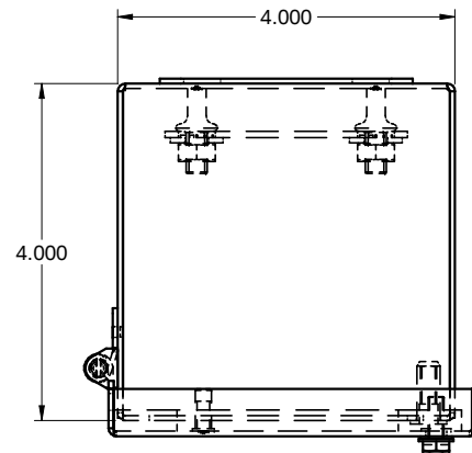
TOP / DESSUS
