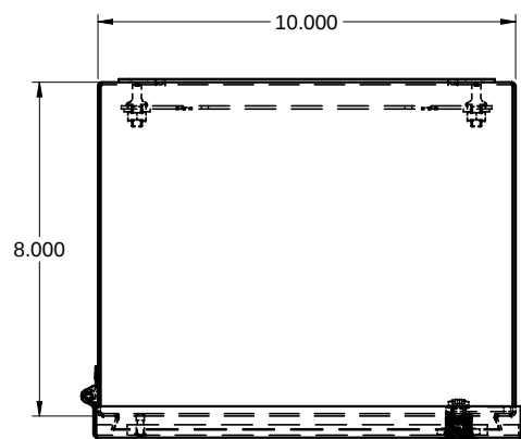
TOP / DESSUS
