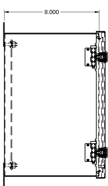
SIDE / CÔTÉ
