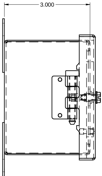
SIDE / CÔTÉ
