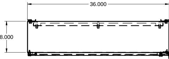
TOP / DESSUS
