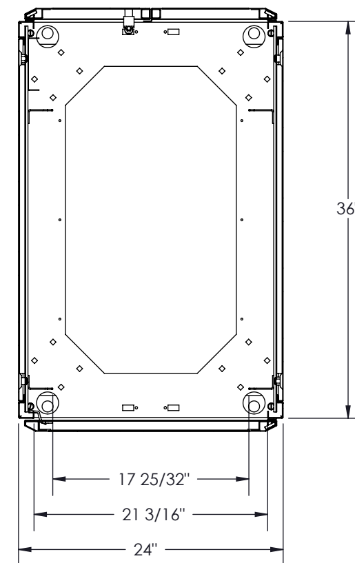
SECTION D-D
