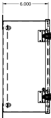
SIDE / CÔTÉ
