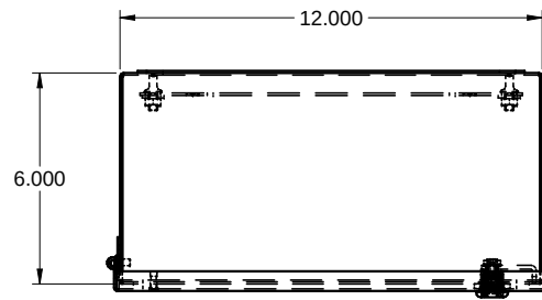
TOP / DESSUS
