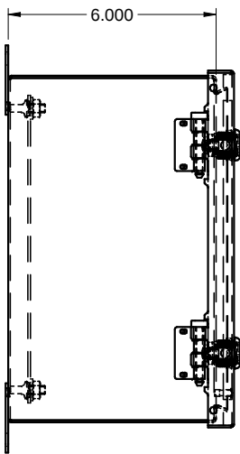
SIDE / CÔTÉ
