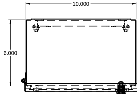
TOP / DESSUS
