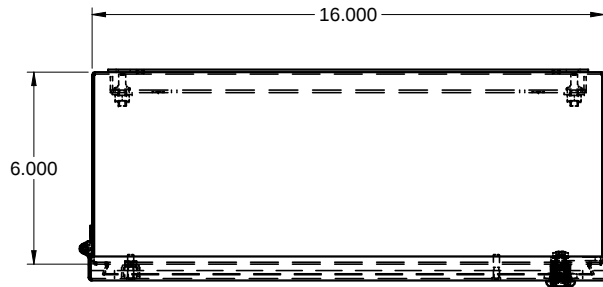
TOP / DESSUS
