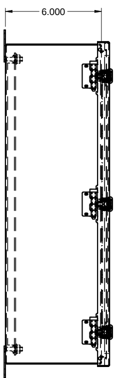
SIDE / CÔTÉ
