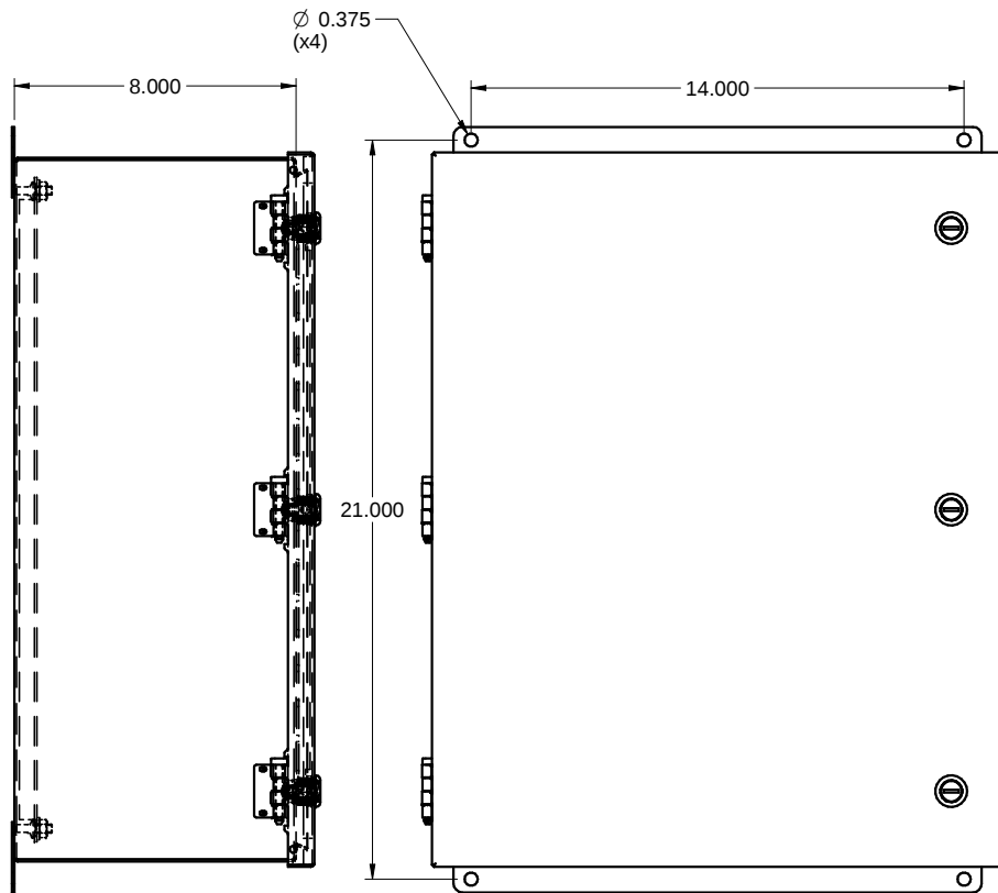
SIDE / CÔTÉ
